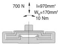
Carichi dinamici max. ammissibili per Drylin® N
