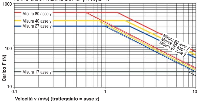
Carichi dinamici max. ammissibili per Drylin® N
